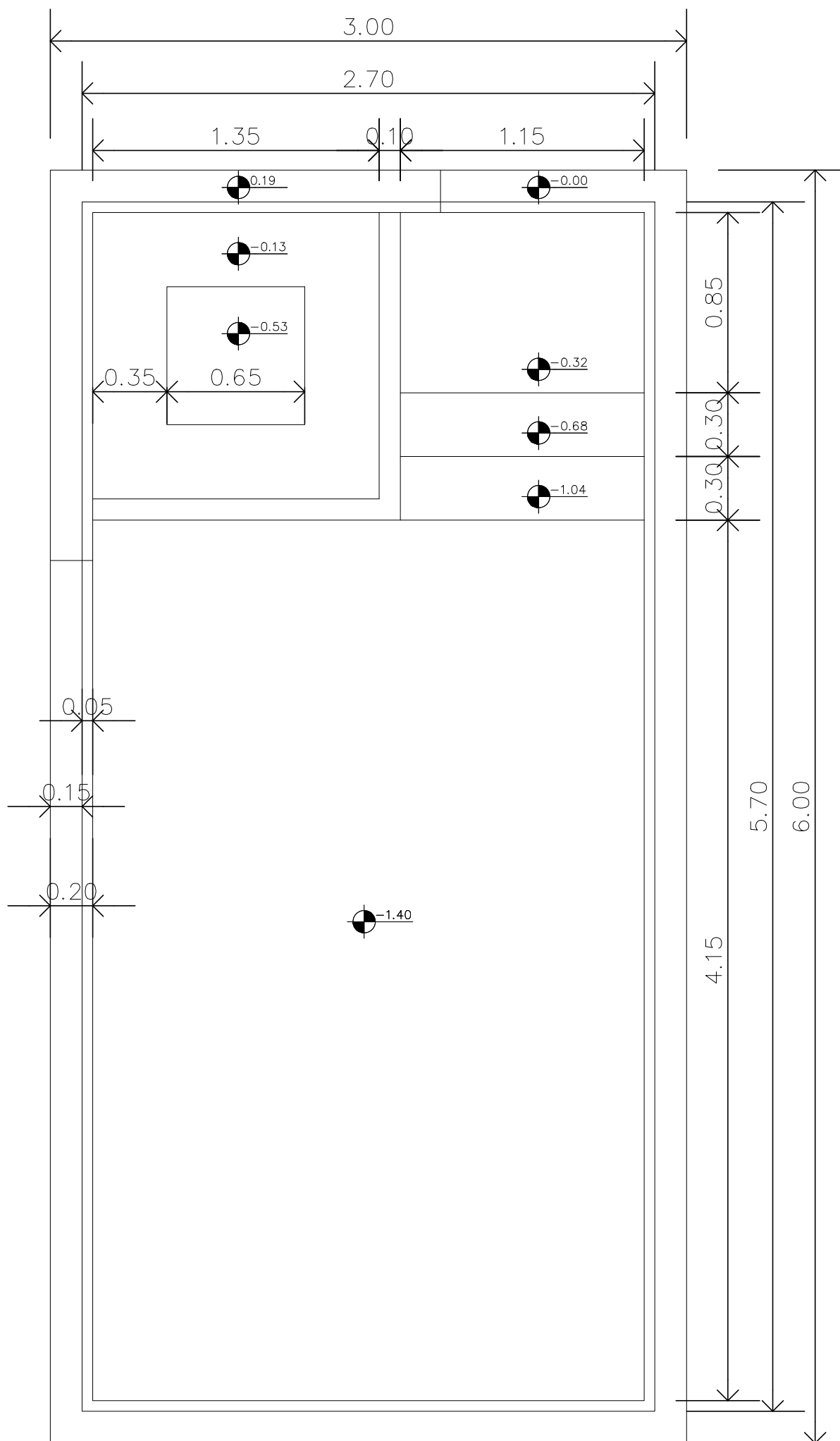
PLANTA BAIXA (6.00x3.00)
